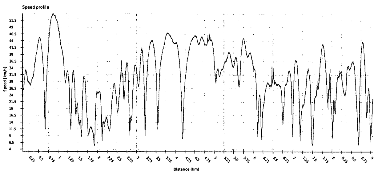
FIGURA 100 VARIAȚIA VITEZEI DE-A LUNGUL LINIEI 11 SENS ORTELEC – BRĂDET
