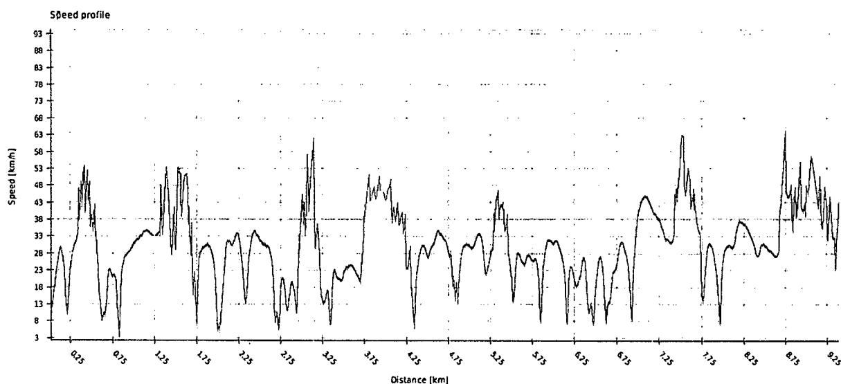
FIGURA 103 VARIAȚIA VITEZEI DE-A LUNGUL LINIEI 22 SENS BRĂDET – GARA ZALĂU
