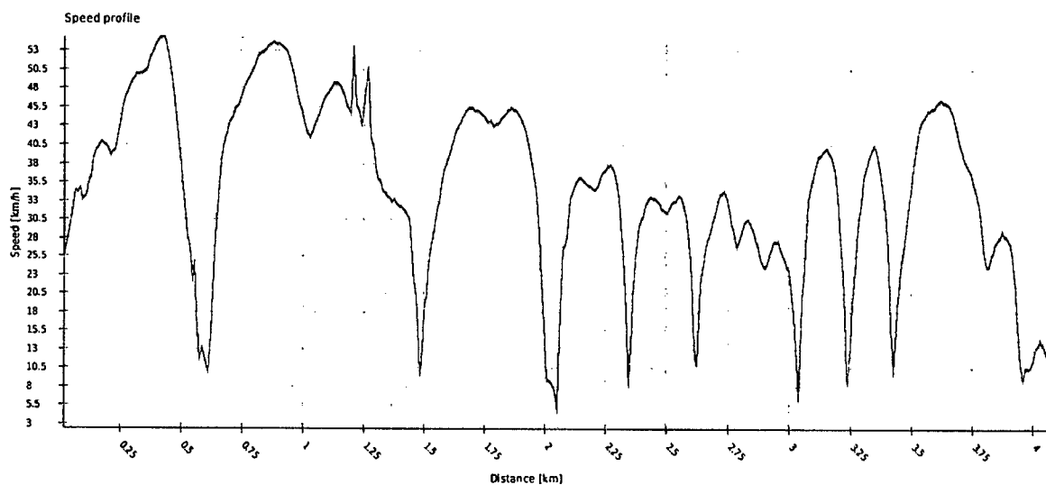
FIGURA 102 VARIAȚIA VITEZEI DE-A LUNGUL LINIEI 13 SENS SĂRMAȘ – CENTRU
