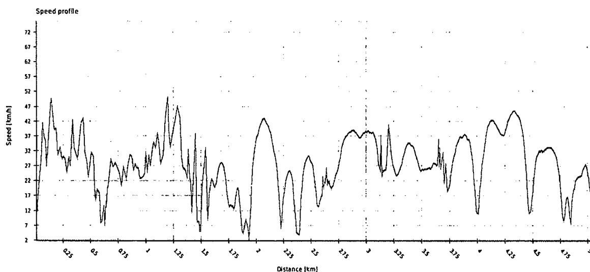
FIGURA 97 VARIAȚIA VITEZEI DE-A LUNGUL LINIEI 4 SENS BRĂDET – DUMBRAVA NORD
