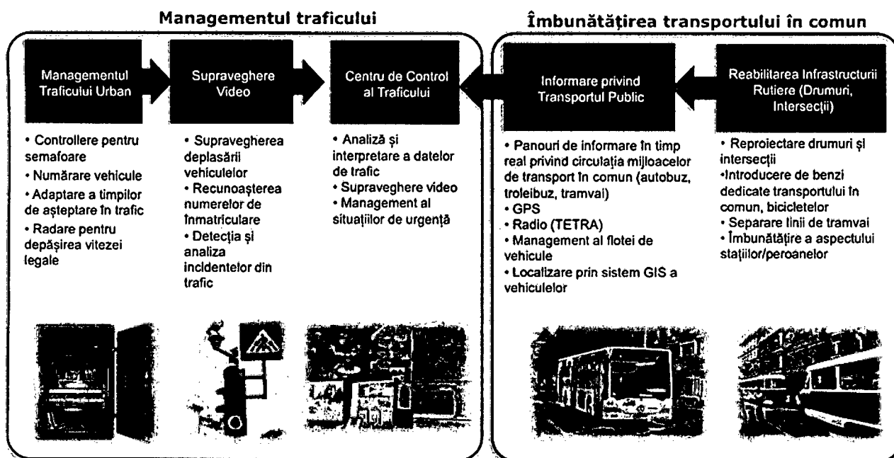
FIGURA 177 ARHITECTURA UNUI SISTEM DE MANAGEMENT AL TRAFICULUI
