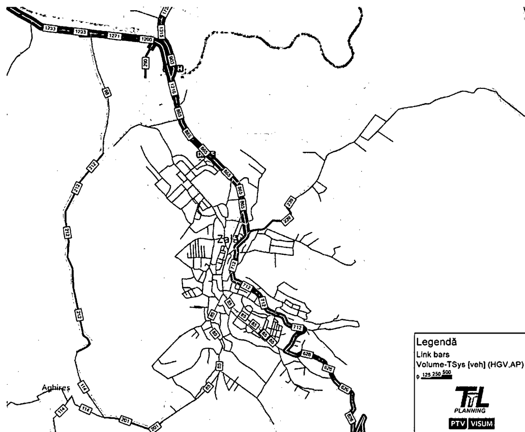
FIGURA 115 NIVELUL DE SERVICIU AL REȚELEI RUTIERE – AN DE BAZĂ 2020
