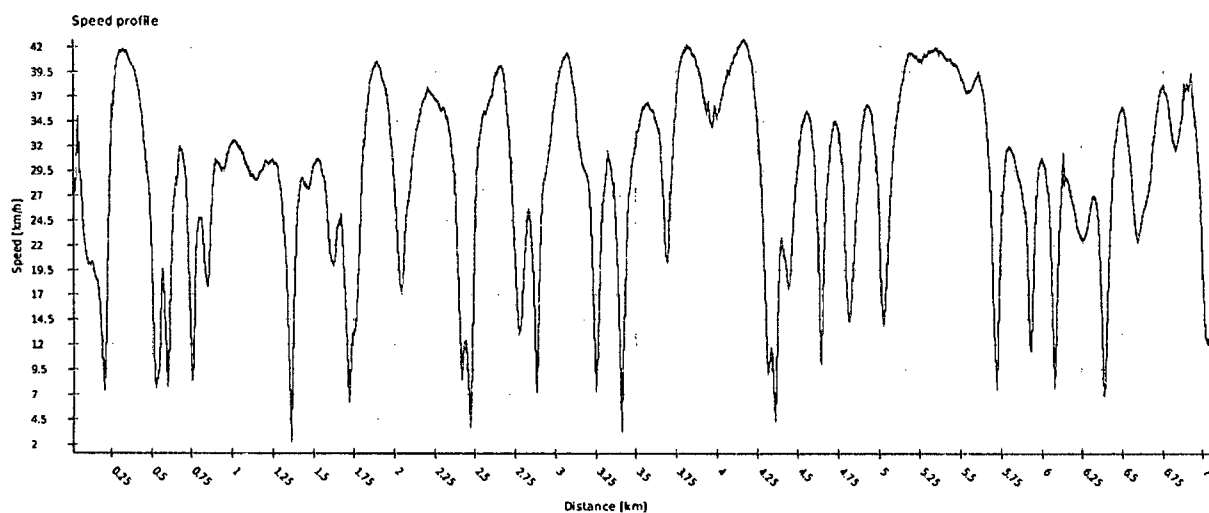
FIGURA 93 VARIAȚIA VITEZEI DE-A LUNGUL LINIEI 1 SENS BRĂDET – GARA ZALĂU
