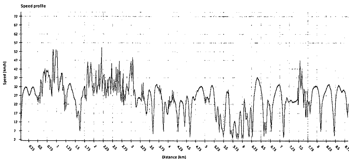
FIGURA 104 VARIAȚIA VITEZEI DE-A LUNGUL LINIEI 22 SENS GARA ZALĂU – BRĂDET
