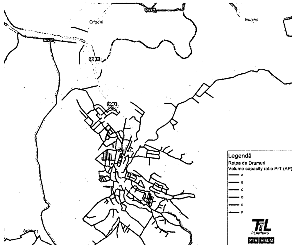
FIGURA 115 NIVELUL DE SERVICIU AL REȚELEI RUTIERE – AN DE BAZĂ 2020
