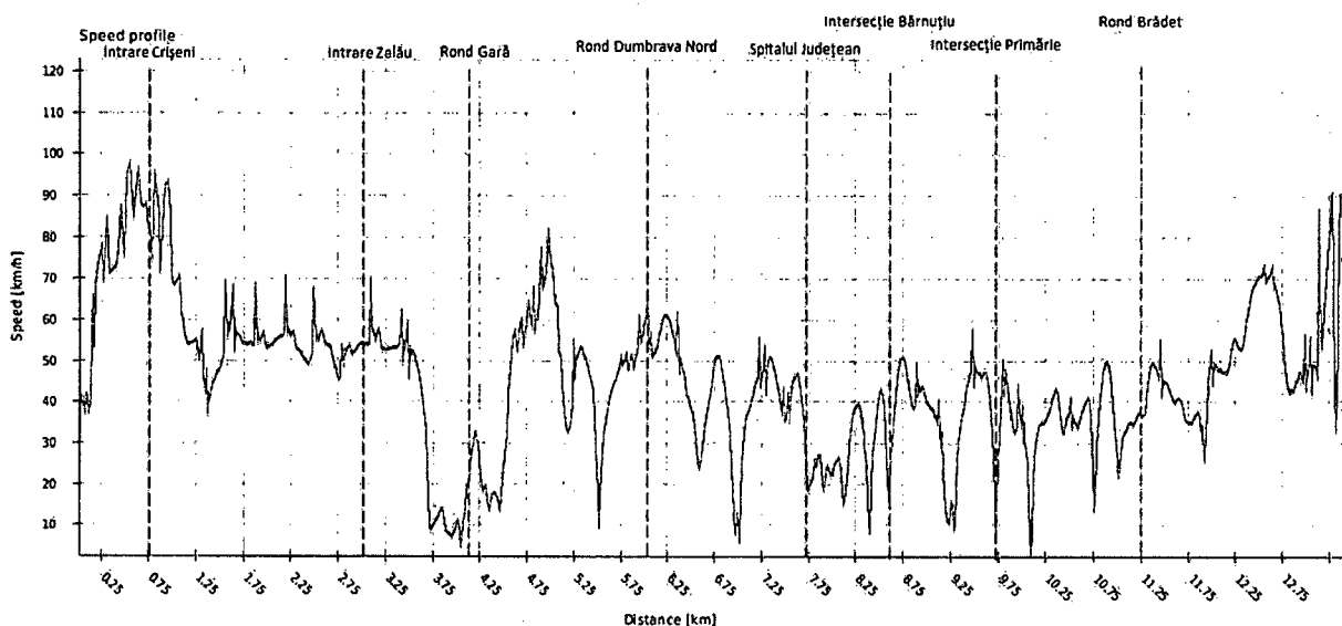
FIGURA 91 VARIAȚIA VITEZEI DE-A LUNGUL TRASEULUI 3 (VERDE) SENS CRIȘENI - MESEȘ
