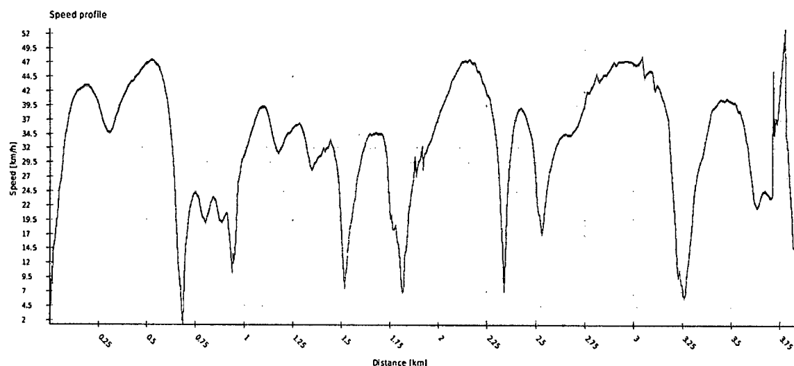
FIGURA 101 VARIAȚIA VITEZEI DE-A LUNGUL LINIEI 13 SENS CENTRU – SĂRMAȘ
