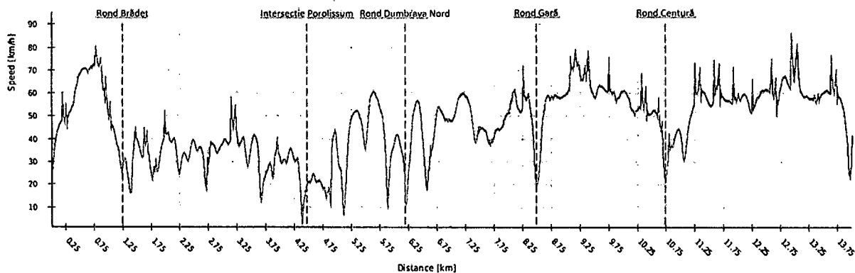
FIGURA 86 VARIAȚIA VITEZEI DE-A LUNGUL TRASEULUI 1 (ALBASTRU) SENS MESEȘ - HERECLEAN
