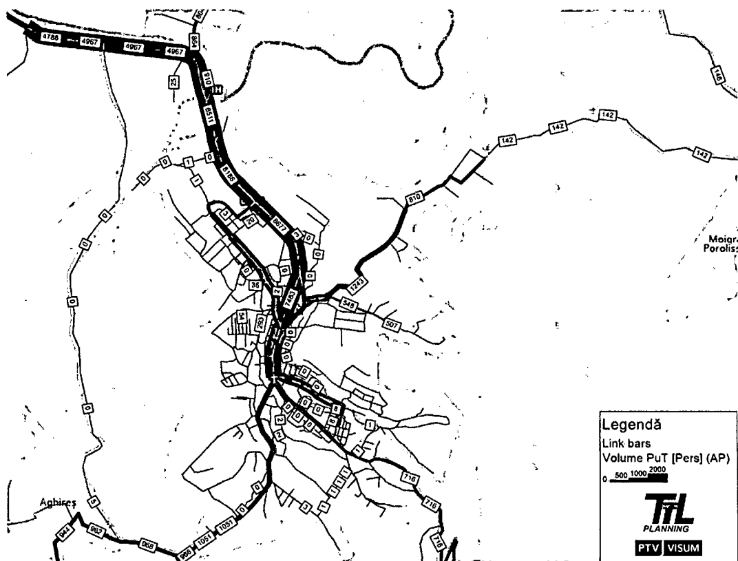
FIGURA 143 SCENARIUL MINIM - MĂRIMEA FLUXURILOR DE TRAFIC – TRANSPORT PUBLIC
