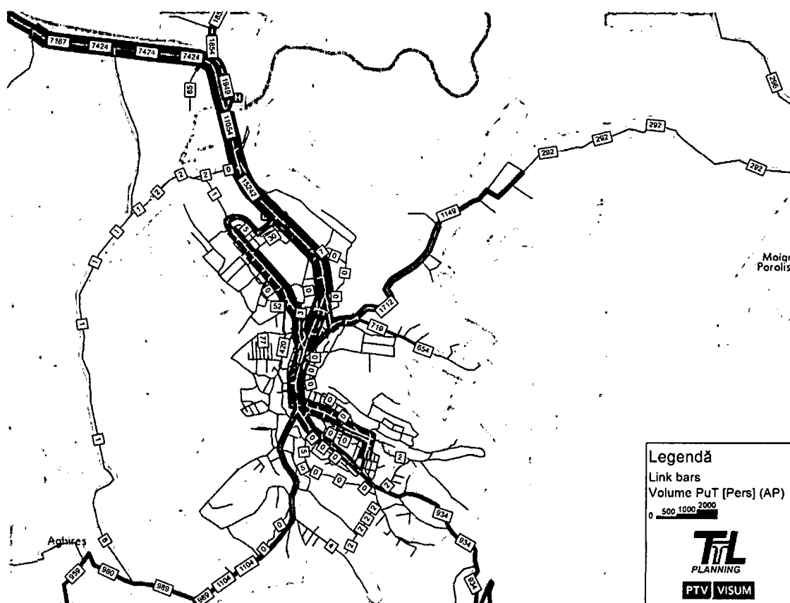
FIGURA 148 SCENARIUL MEDIU - MĂRIMEA FLUXURILOR DE TRAFIC – TRANSPORT PUBLIC
