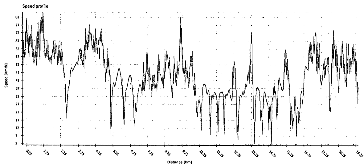
FIGURA 96 VARIAȚIA VITEZEI DE-A LUNGUL LINIEI 2 SENS VALEA MIȚII – GARA ZALĂU
