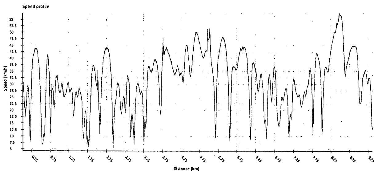
FIGURA 99 VARIAȚIA VITEZEI DE-A LUNGUL LINIEI 11 SENS BRĂDET – ORTELEC
