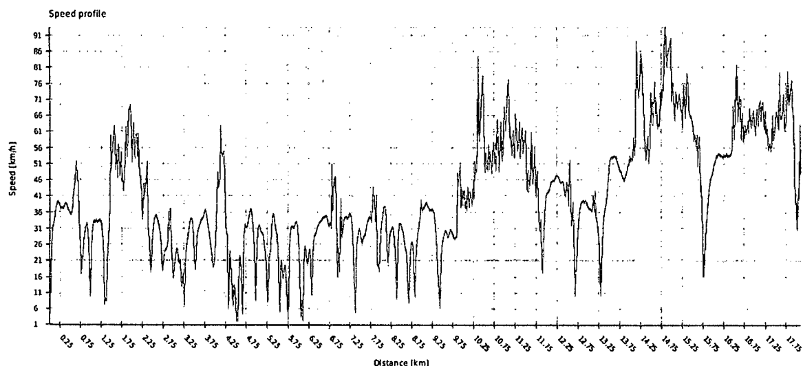
FIGURA 95 VARIAȚIA VITEZEI DE-A LUNGUL LINIEI 2 SENS GARA ZALĂU – VALEA MIȚII
