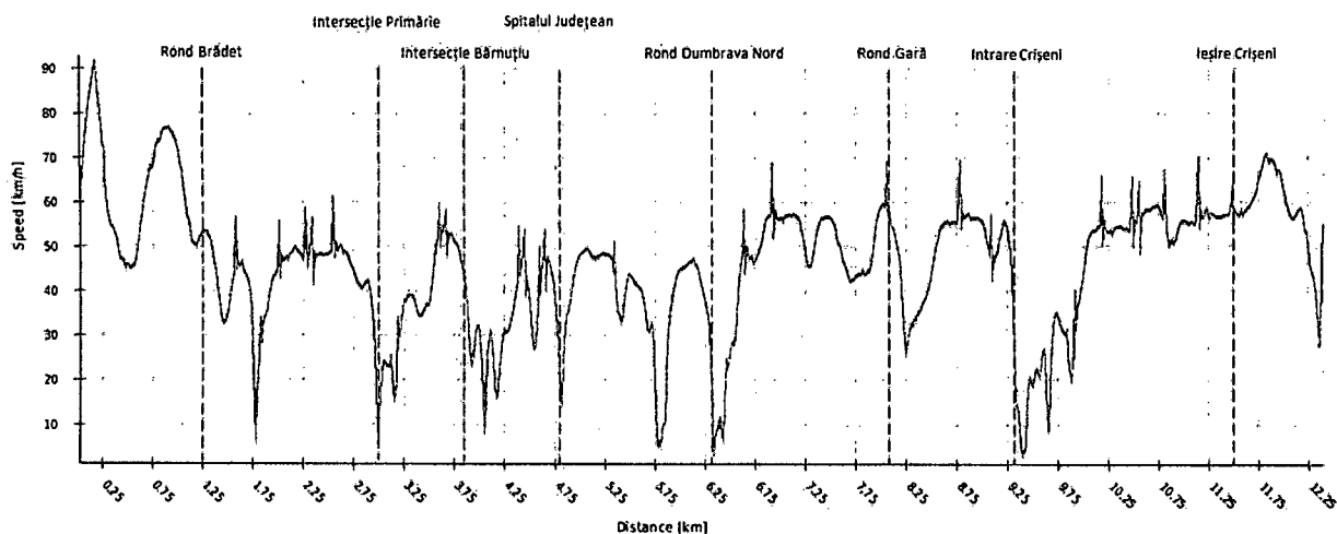
FIGURA 90 VARIAȚIA VITEZEI DE-A LUNGUL TRASEULUI 3 (VERDE) SENS MESEȘ - CRIȘENI
